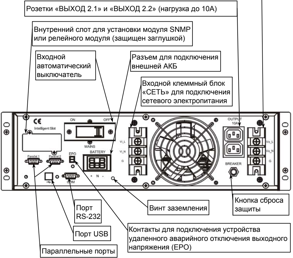
Рисунок 2 — Общий вид задней панели изделия со снятыми защитными крышками
